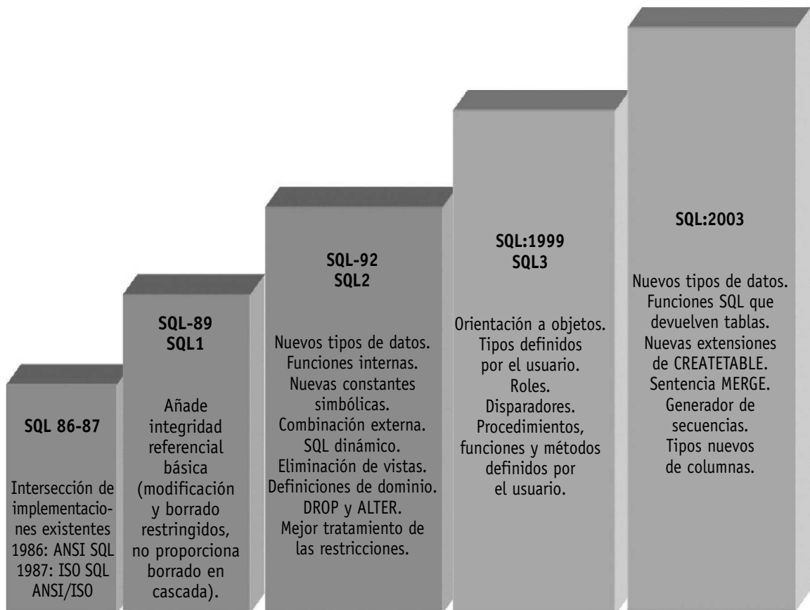
Figura 3.2. Estándares SQL.
