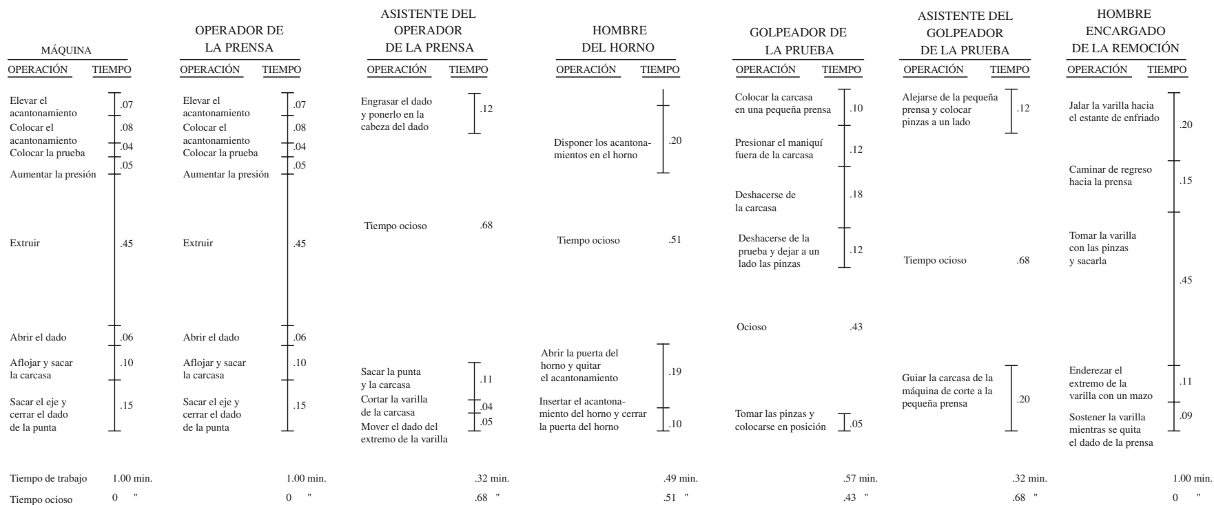
DIAGRAMA DE PROCESOS DE GRUPO DEL MÉTODO ACTUAL Extrusión hidráulica Departamento de prensado II Planta de Bellefonte, Pa. Dibujado por B.W.N. 4-15- Diagrama núm. G-85
