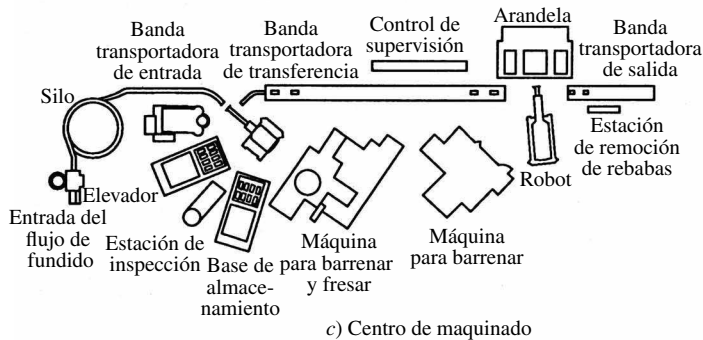
Figura 3.9 Dibujo que ilustra algunas de las aplicaciones industriales más comunes de los robots.
