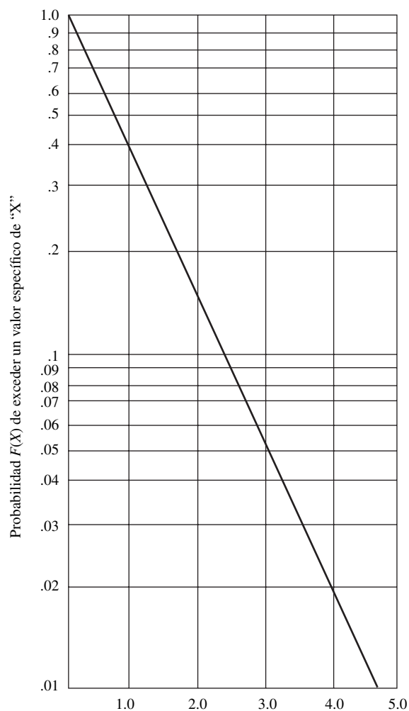
Figura 15.2 Distribución exponencial.
