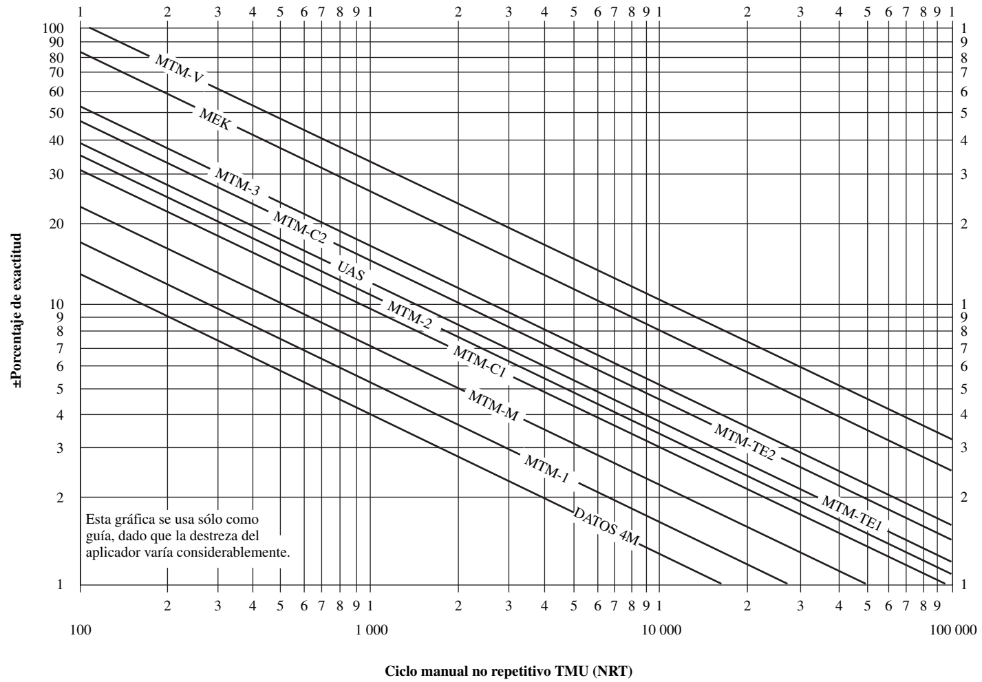
Figura 13.10 Exactitud absoluta total a un nivel de confianza de 90% de los diferentes sistemas MTM.
