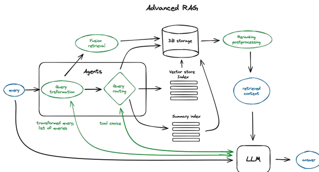
Figura 11. Diagrama esquemático del flujo del Advanced RAG.
