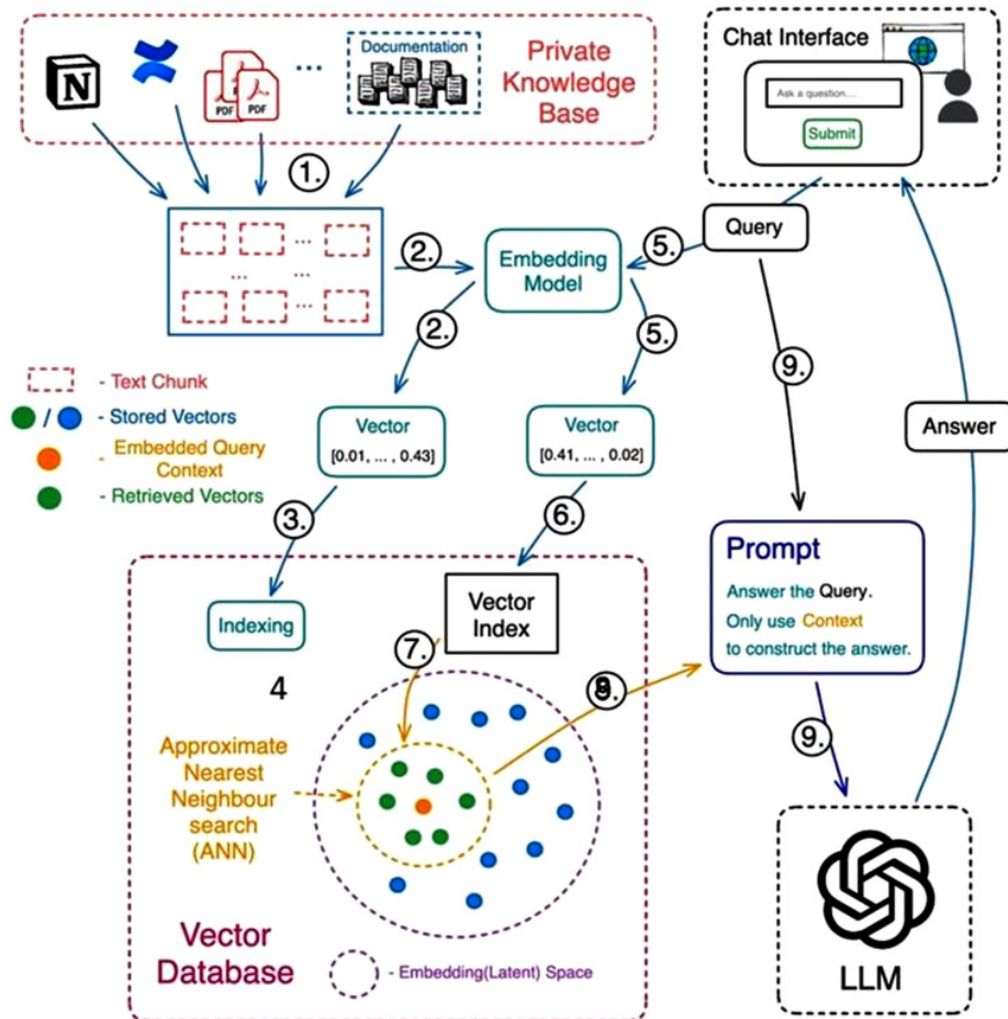
Fig. 5. Diagrama general que ilustra el flujo de integración entre el módulo de recuperación y el módulo de generación. Tomado de: https://pica.zhimg.com/v2-48776c054f9bc2c65a118ff31b0422e6_1440w.jpg
