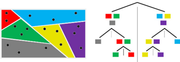
Fig. 8. Ejemplo de la estructuración de datos en árboles para búsquedas eficientes mediante ANNOY. Tomado de: https://360digit.b-cdn.net/assets/admin/ckfinder/userfiles/images/blog/Annoy-in-Python/09%20%20Annoy%20Vector%20database-03.png
