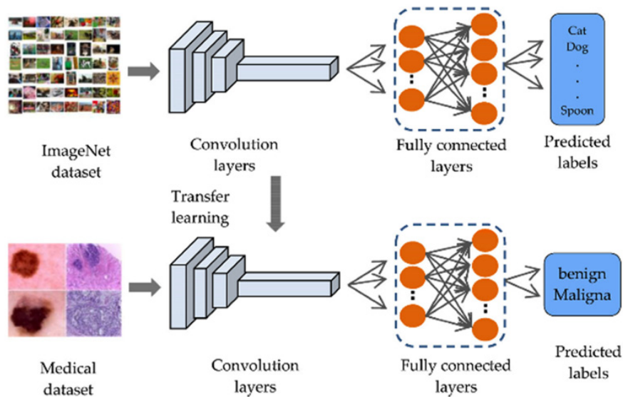
Fig. 4. Ejemplo de integración de información a partir de modelos generativos en aplicaciones prácticas. Tomado de: https://pub.mdpi-res.com/sensors/sensors-23-00570/article_deploy/html/images/sensors-23-00570-g001.png?1672823988
