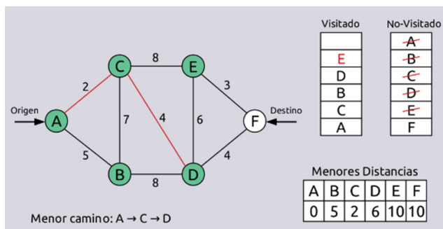
Fig. 9. Ejemplo de visualización de la conectividad y caminos en un grafo mediante el algoritmo de Dijkstra. Tomado de: https://raw.githubusercontent.com/the-akira/PythonExperimentos/master/Algoritmos/Dijkstra/Imagens/Grafo7.png
