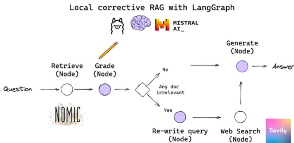
Fig. 10. Diagrama del flujo de trabajo en el Corrective RAG. Tomado de: https://i.ytimg.com/vi/E2shqsYwxck/maxresdefault.jpg
