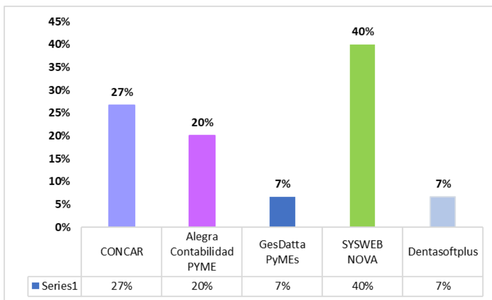
Software implementado
