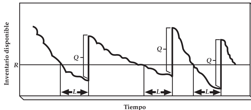
FIGURA 15.7 Sistema de revisión continua.
