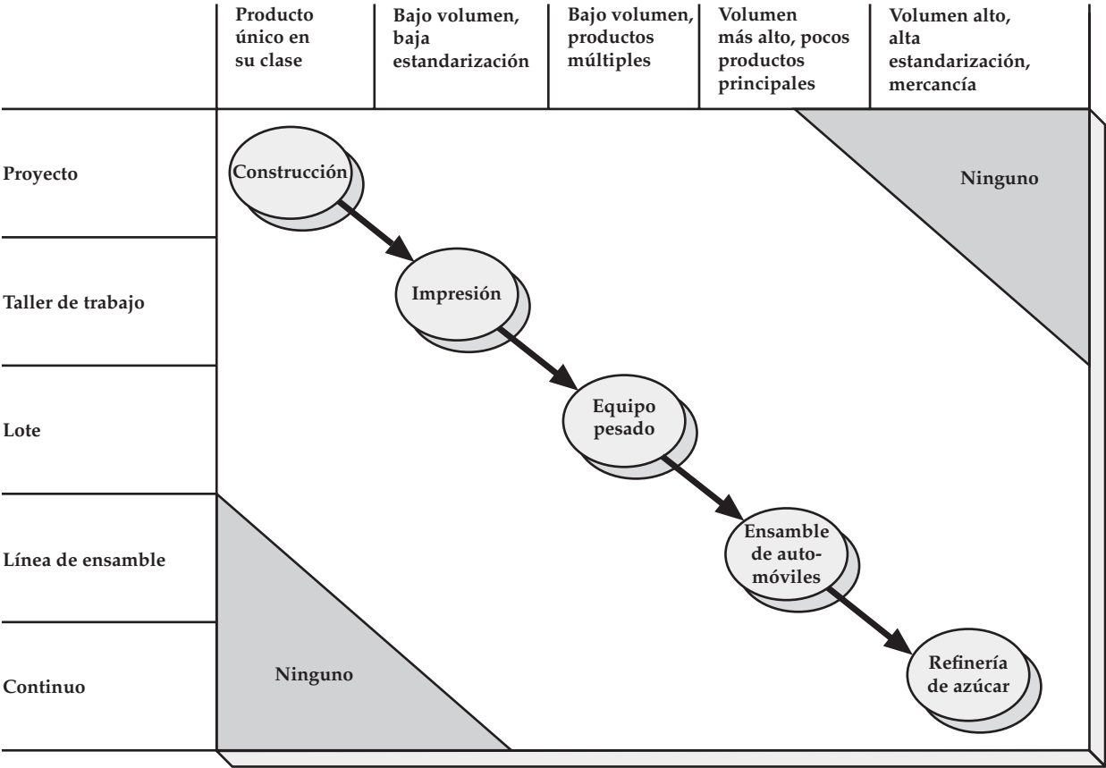
FIGURA 4.5 Matriz producto-proceso.
