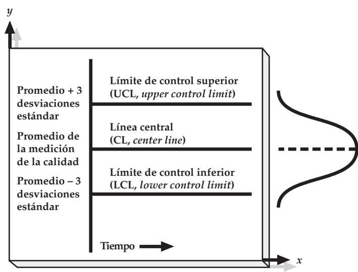
FIGURA 9.1 Gráfica de control de calidad.
